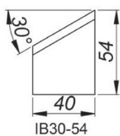
30° Beitelplaat binnenzijde afschuiven, Hoogte 54 mm [IB30/54] Product Code: NOZ-000025
