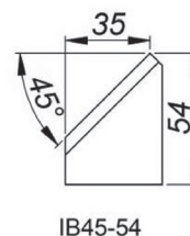
45° Beitelplaat binnenzijde afschuiven, Hoogte 54 mm [IB45/54] Product Code: NOZ-000026
