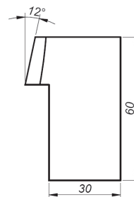
12° Speciaal gereedschap Hoogte 60 mm Product Code: NOZ-000086
