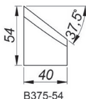
37.5° Beitelplaat buitenzijde afschuiven, Hoogte 54 mm [B375/54] Product Code: NOZ-000015
