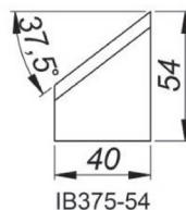
37.5° Beitelplaat binnenzijde afschuiven, Hoogte 54 mm [IB375/54] Product Code: NOZ-000024
