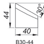
30° Beitelplaat buitenzijde afschuiven, Hoogte 44 mm [B30/44] Product Code: NOZ-000018
