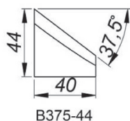
37.5° Beitelplaat buitenzijde afschuiven, Hoogte 44 mm [B375/44] Product Code: NOZ-000020
