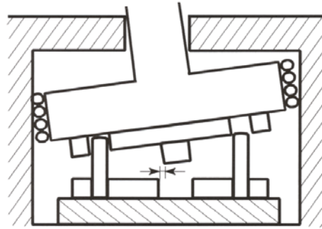
figuur 4.8 Door verkanting van de stoter ontstaan er centreringsfouten
