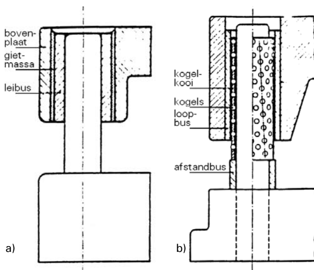
figuur 4.5 Bus- versus kogelgeleiding
