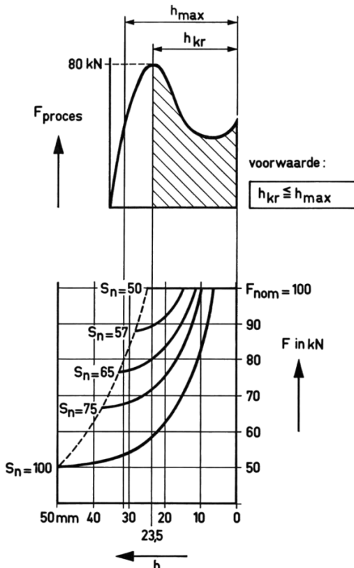
figuur 3.4 Maximale kracht "F" op een afstand "h" vóór het onderste dode punt bij verschillende slaginstellingen van een excenterpers
