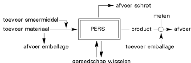
figuur 3.1 De fysieke stromen rond de pers
