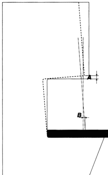
figuur 3.11 Asymmetrisch veergedrag van een C-framepers bij een dynamische belasting van 500 kN. A = 0,672 mm; B = 0,48 mm
