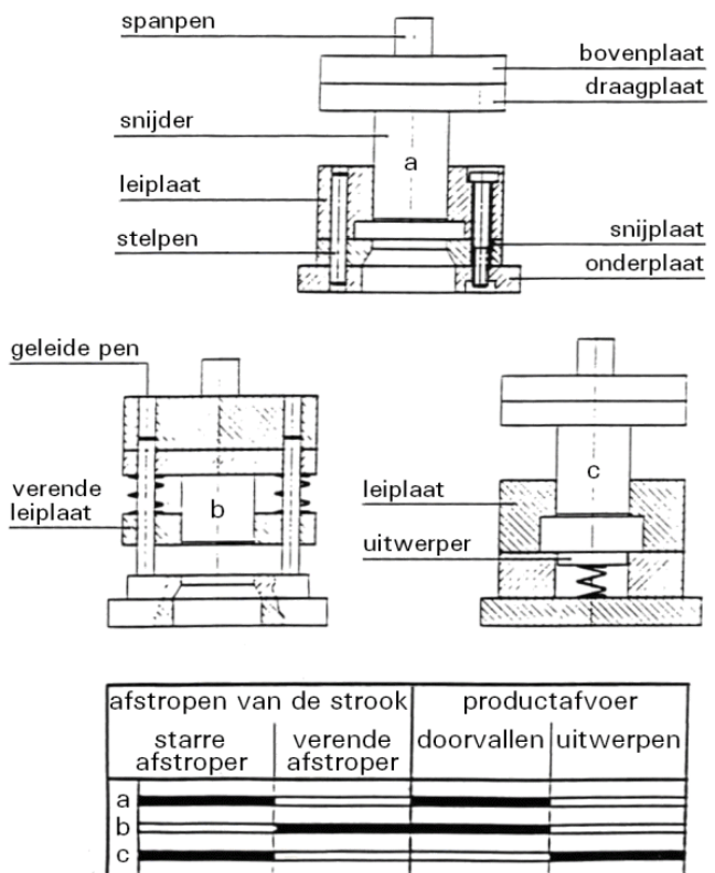
figuur 4.2 Ponsgereedschappen met vaste leiplaat en met geleidezuilen
