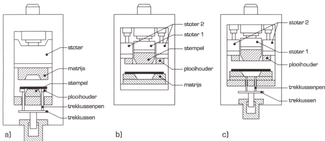
figuur 3.9 Drievoudig werkende pers met onderliggende (a) en bovenliggende (b en c) plooihouder
