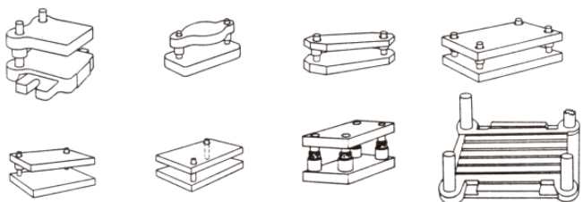
figuur 4.3 In de handel verkrijgbare stempelhuizen [lit.2]
