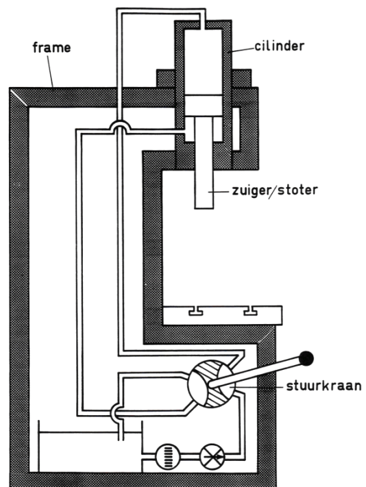
figuur 3.6 Hydraulische pers
