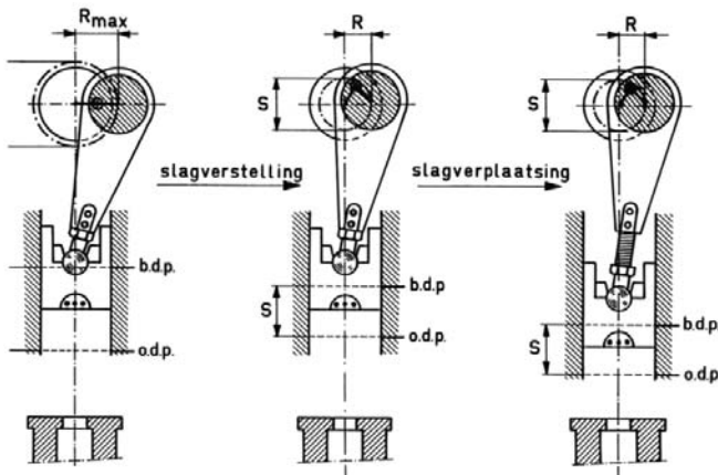
figuur 3.3 Correctie onderste dode punt na slagverstelling
